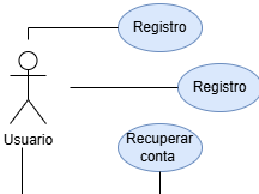
diagrama 1 - Login
