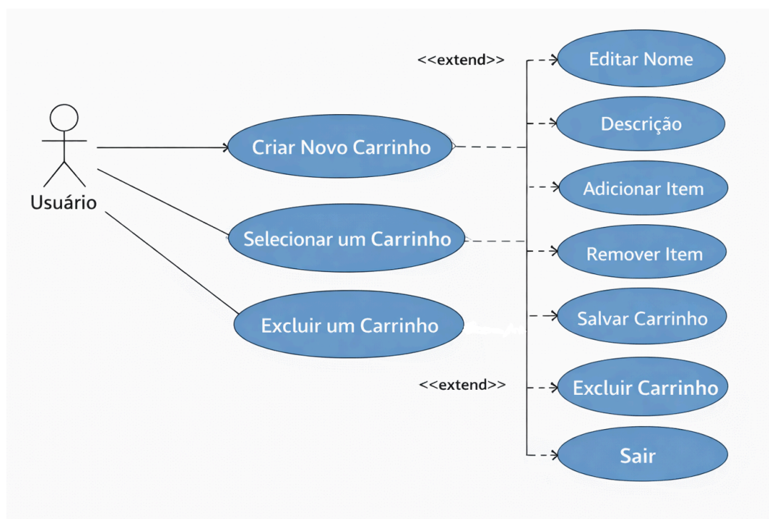
Diagrama 3 - carrinho
